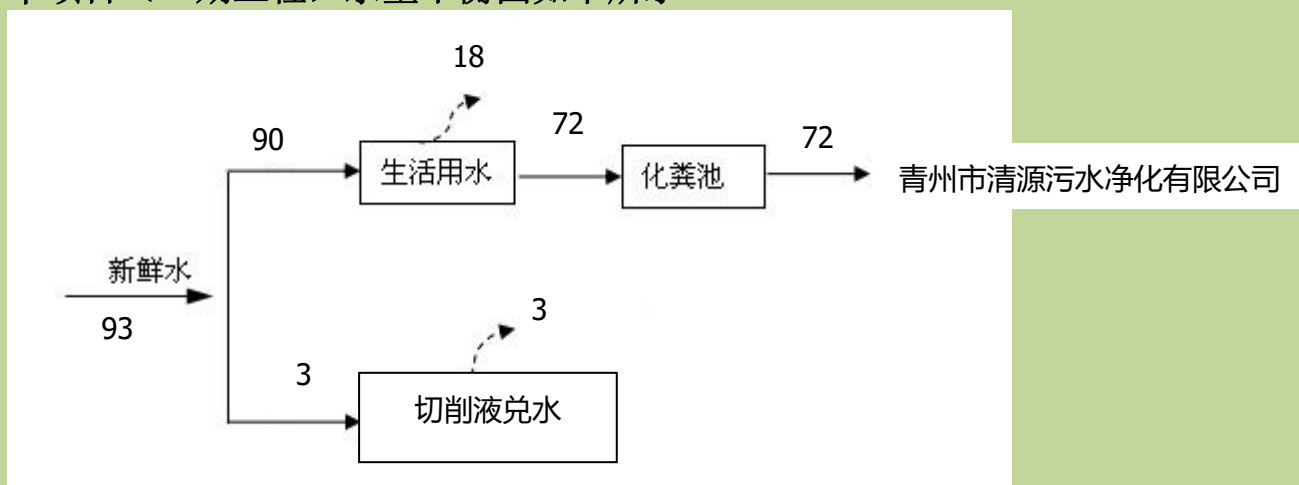
项目（一期工程）水量平衡图（单位：t/a）
